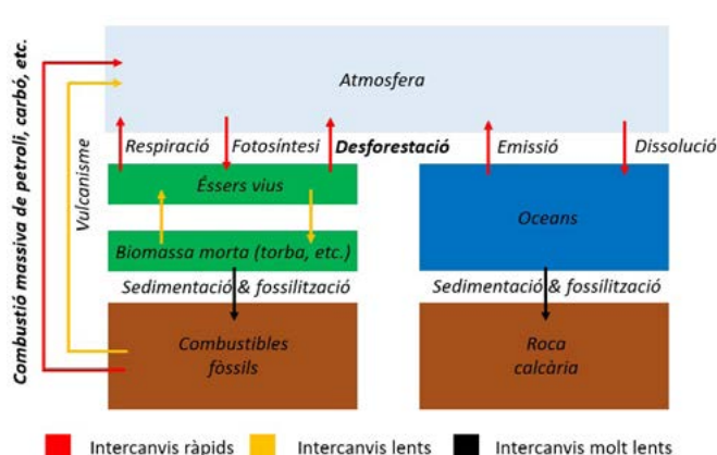
Figura 5: Intercanvis entre els diferents reservoris de Carboni
