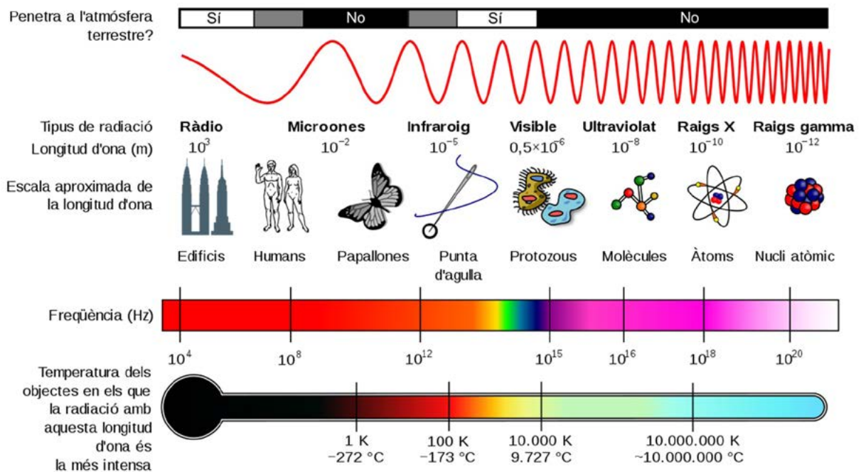
Figura 1: Espectre electromagnètic
