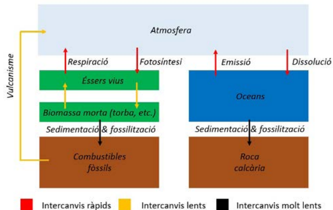
Figura 4: Intercanvis naturals entre els diferents reservoris de Carboni
