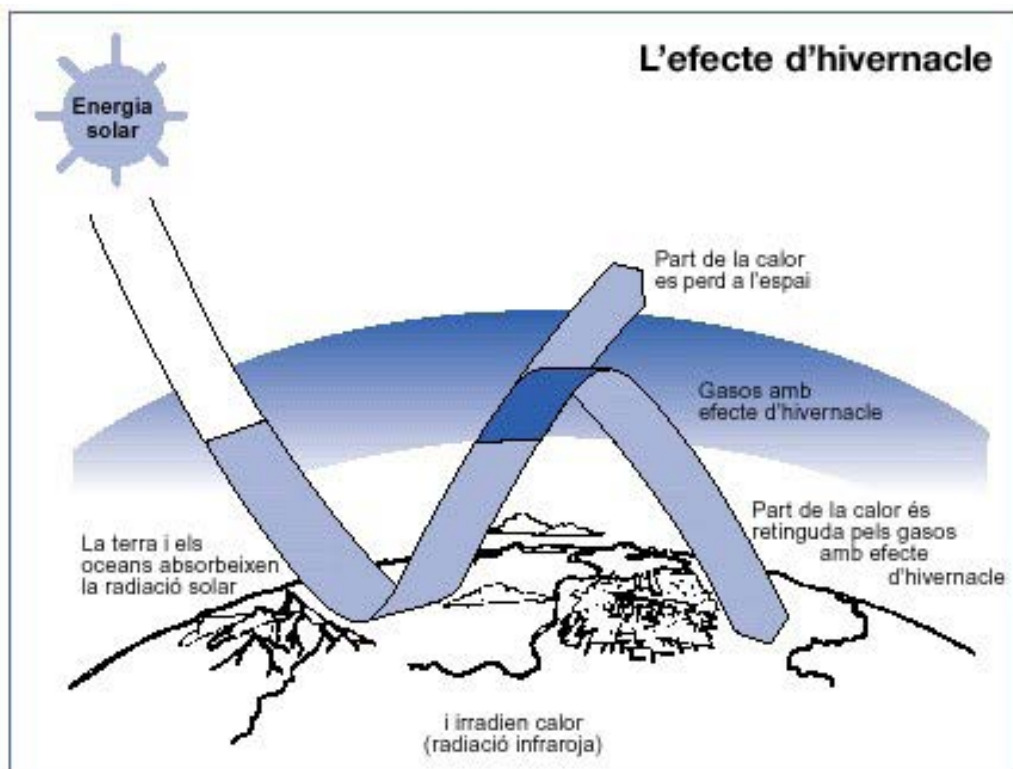
Figura 2: Influència dels gasos amb efecte hivernacle
