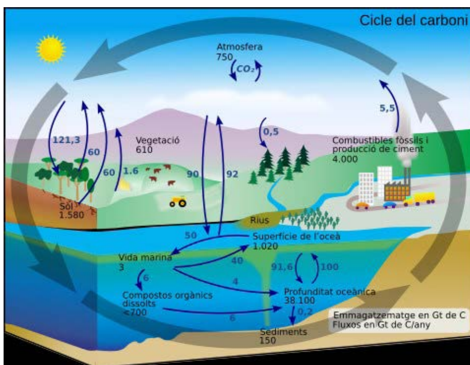
Figura 3: Cicle del carboni en el planeta Terra (Gt significa GigaTones)
