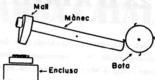
Esquema del martinet
